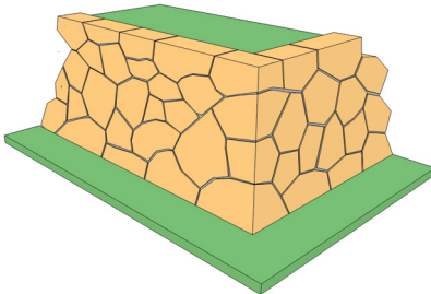
Bild 3: Hammerrechtes Zyklopenmauerwerk (Quelle: Diebel, Meier, Hübner)
